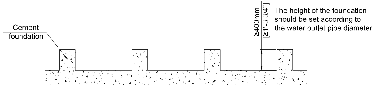
SECTION A-A
