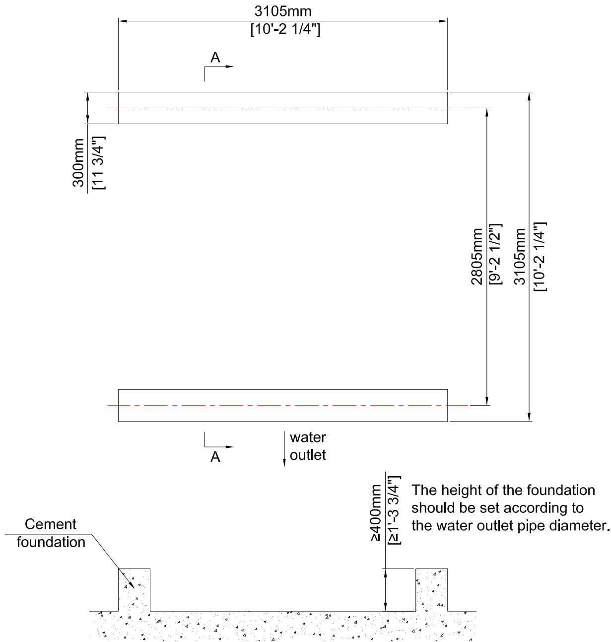
SECTION A-A
